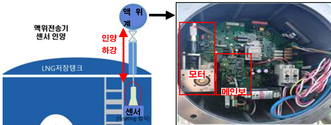
【그림】 LNG 저장탱크 액위계 개요 및 주요부품
